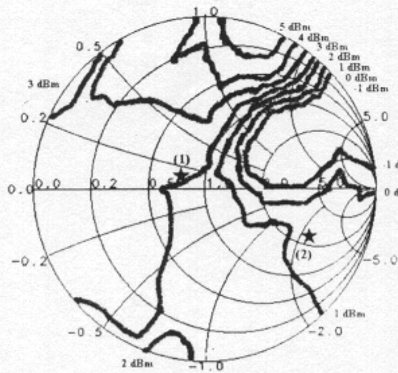
그림 8. 입력 전력이 -4 dBm일 때 2차 하모닉의 제적. 표준 증폭기의 출력 정합 회로의 2F_0 에서의 입력 임피던스(별표 (1)), 그리고 소형화된 증폭기의 출력 정합 회로의 2F_0 에서의 입력 임피던스(별표 (2))
