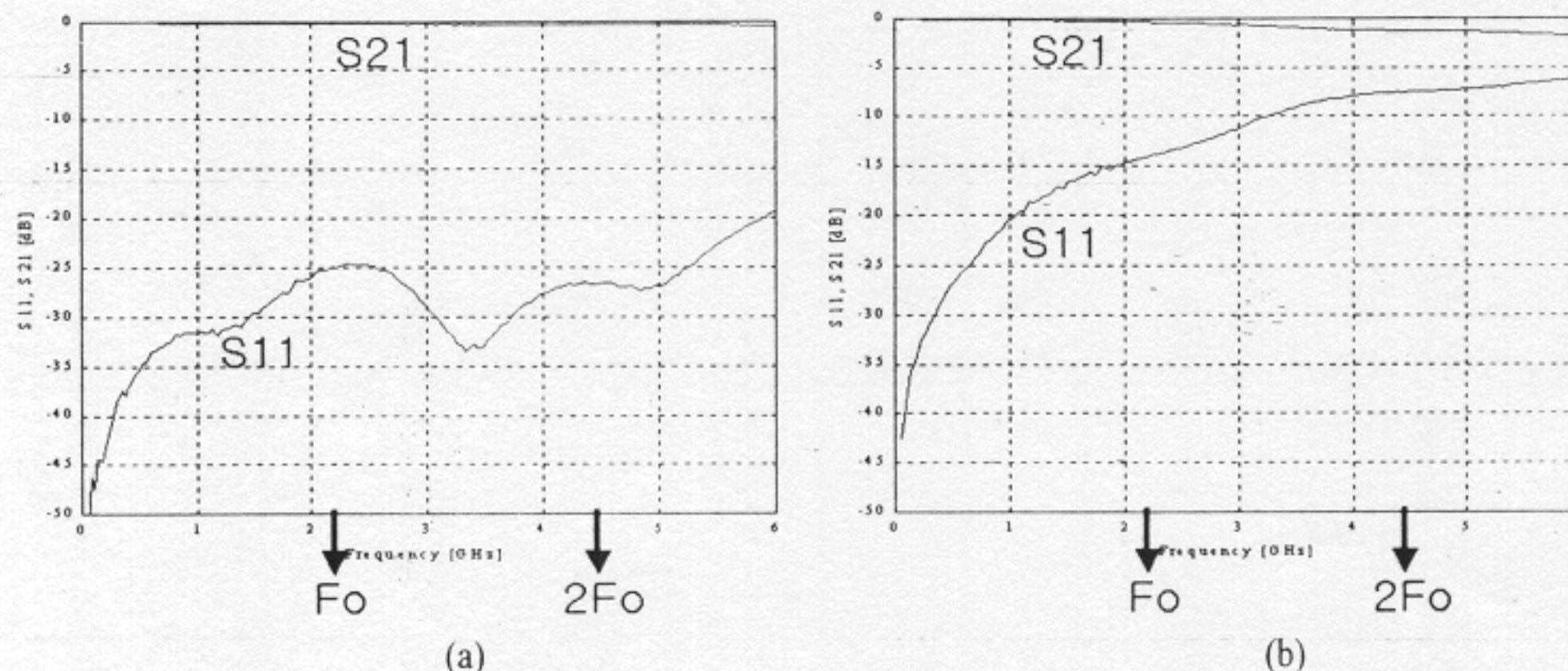
그림 6. 그림 4에서 길이가 (a) 길이가 L_2 인 표준형 마이크로스트립 선로와 (b) 길이가 L_2' 인 DGS 선로의 측정된 전달 특성
