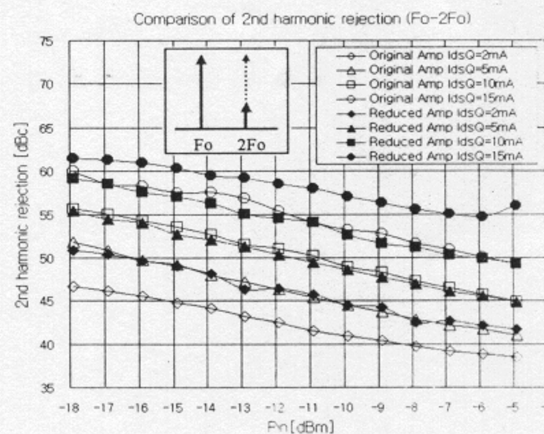
그림 7. 두 증폭기의 측정된 2차 하모닉 차단 특성 ( F_0-2F_0 )
