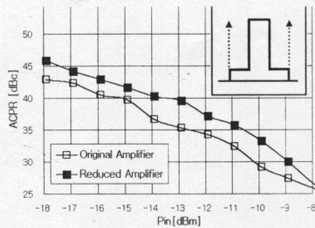
그림 10. 측정된 ACPR 특성( I_{dsQ}=10\text{ mA} ) Fig. 10. Comparison of the measured ACPR( I_{dsQ}=10\text{ mA} ).
