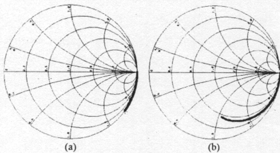
그림 3. (a) 표준형 마이크로스트립 선로 2 mm에 대한 S_{21} 위상, (b) 그림 1의 DGS가 결합된 마이크로스트립 선로 2 mm에 대한 S_{21} 위상 (~10 GHz) Fig. 3. S_{21} phases of the (a) standard microstrip line, length 2 mm and (b) microstrip line with the unit DGS and length 2 mm shown in Fig. 1 (~10 GHz).
