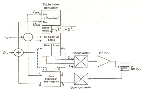
[그림 10] 고정 이득 디지털 전치왜곡 증폭기
