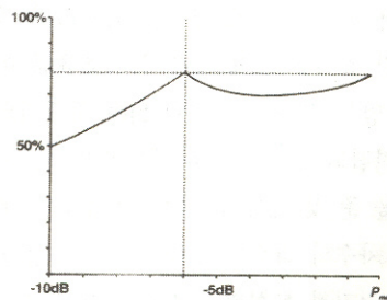
[그림 3] Doherty 증폭기의 효율 특성
