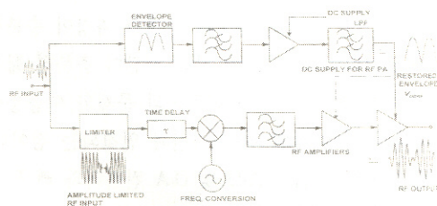
[그림 11] 포락선 제거 및 복원 방식의 블록도
