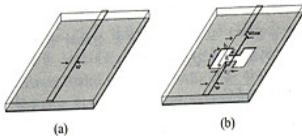
그림 3. (a) 일반적인 마이크로스트립 전송 선로, (b) DGS 마이크로스트립 전송 선로 Fig. 3. (a) Conventional microstrip transmission line, (b) DGS microstrip transmission line.
