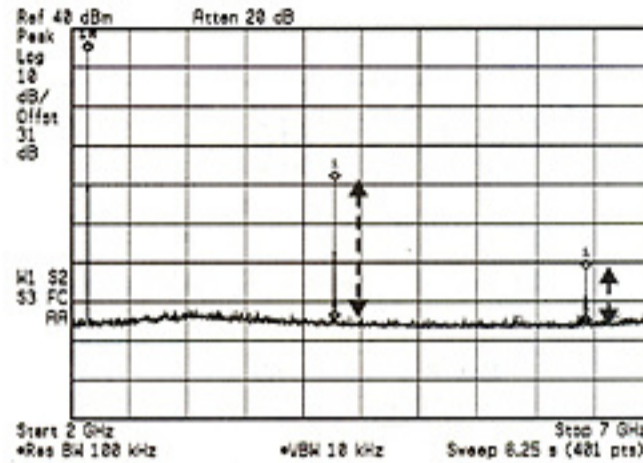
그림 10. 일반적인 주 증폭기와 DGS 주 증폭기의 출력 스펙트럼 비교(@ P_{out}=35 dBm) Fig. 10. Output spectrum comparison between the conventional and the proposed DGS carrier amplifier(@ P_{out}=35 dBm).
