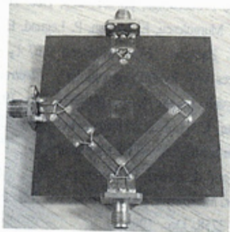
(b) 사각형 레이아웃 (b) Rectangular layout
