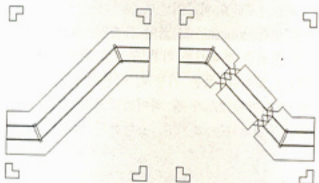
(a) 기준 CPW 전송 선로 (a) Standard CPW line (b) 2개의 180도 위상 반전부가 포함된 CPW 전송 선로 (b) CPW line having 2 cross sections which produce the additional 360° phase
