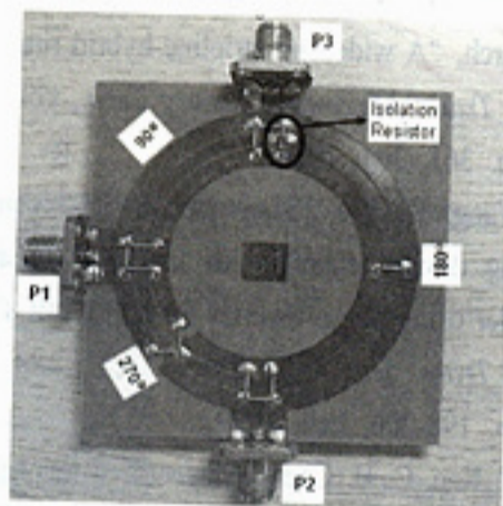
(a) 원형 레이아웃 (a) Circular layout
