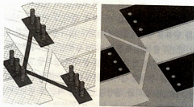
(a) 3차원 투시 그림 (a) 3-dimensional projection (b) CPW 윌킨슨 금속면 레이아웃 (b) CPW metal pattern on the top surface
