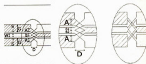
(a) CPW 패턴면 그림 (a) Top view (b) 확대도 (b) Magnified crossing structure (c) 변형된 구조 (c) A modified crossing structure
