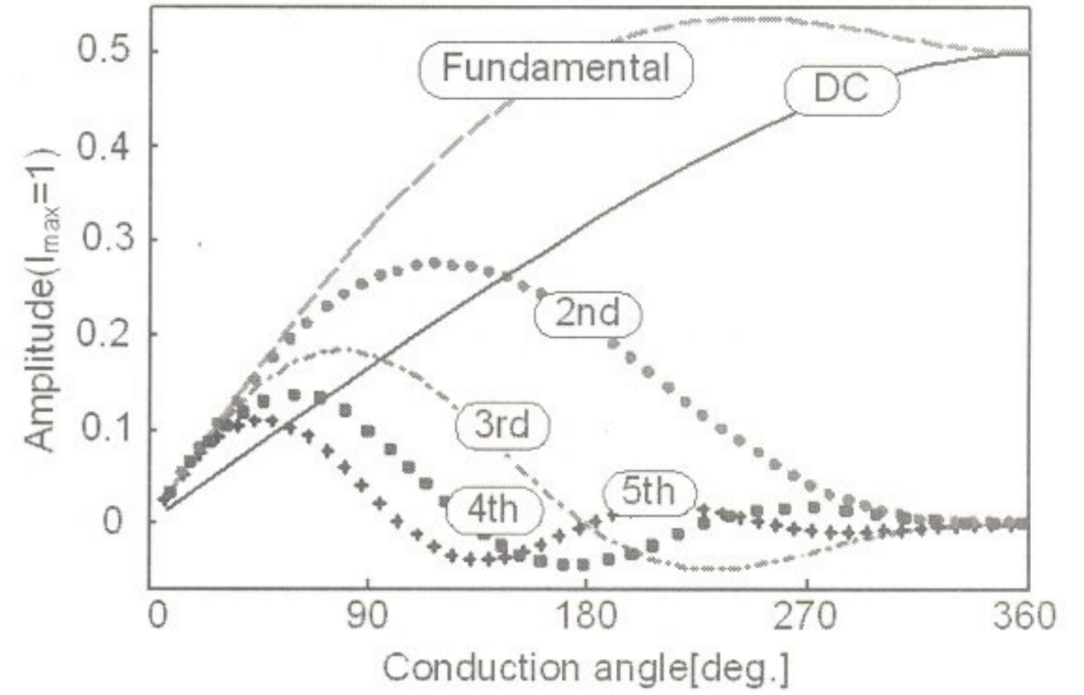
그림 1. 전도각에 따른 기본 신호 성분과 고조파 성분의 크기 비교
