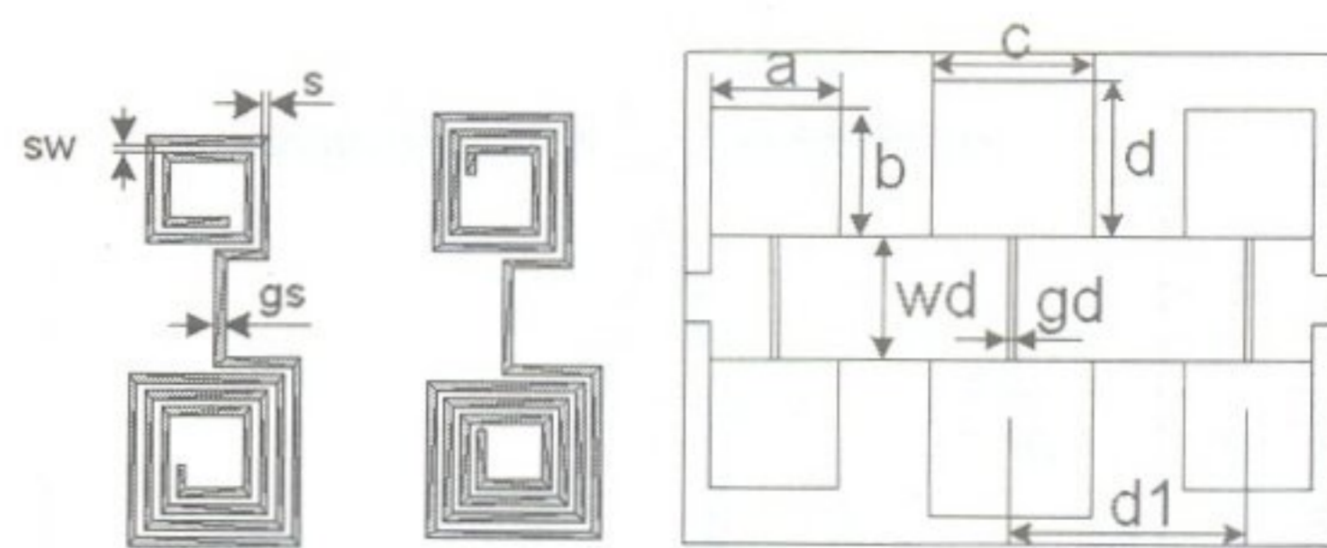
(a) 3체배기의 나선형 단일 DGS (b) 4체배기의 나선형 단일 DGS (c) 2체배기의 아령 DGS (a) Spiral DGS unit for tripler (b) Spiral DGS unit for quadrupler (c) For frequency doubler unit
