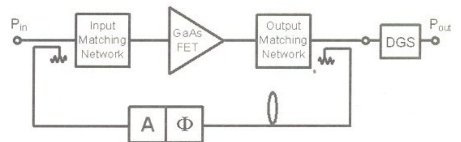
그림 2. 제안된 주파수 체배기의 블록도
