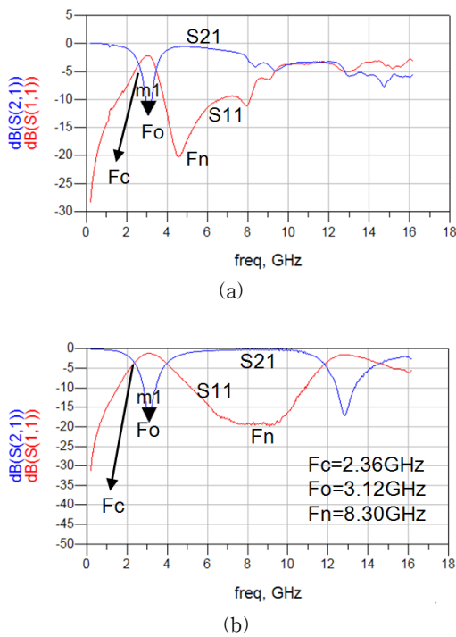
그림 8 제안하는 DL-CRLH 선로의 부분 회로별로 측정된 특성의 예 ( V_r=0V ) (a) 그림 7(a)에 보인 아랫면 회로만 제작하여 측정된 특성 (b) 그림 7(a)에 보인 윗면 회로만 제작하여 측정된 특성
