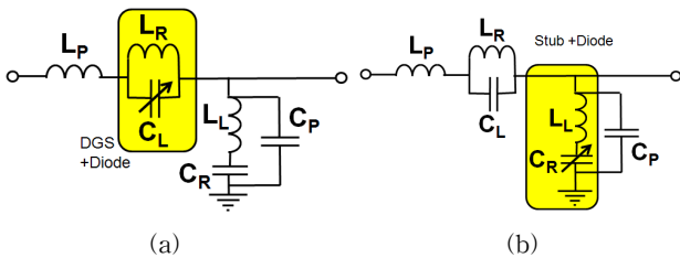
그림 4 주파수 가변성을 갖는 DL-CRLH 전송선로 (a) 직렬 연결된 병렬공진 회로의 C_L 을 가변 (b) 셉트 연결된 직렬공진 회로의 C_R 을 가변
